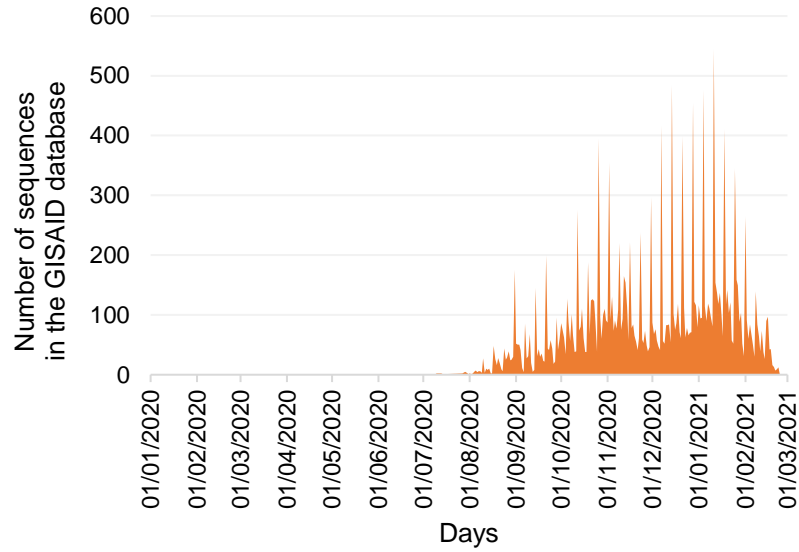
20E (EU1)
