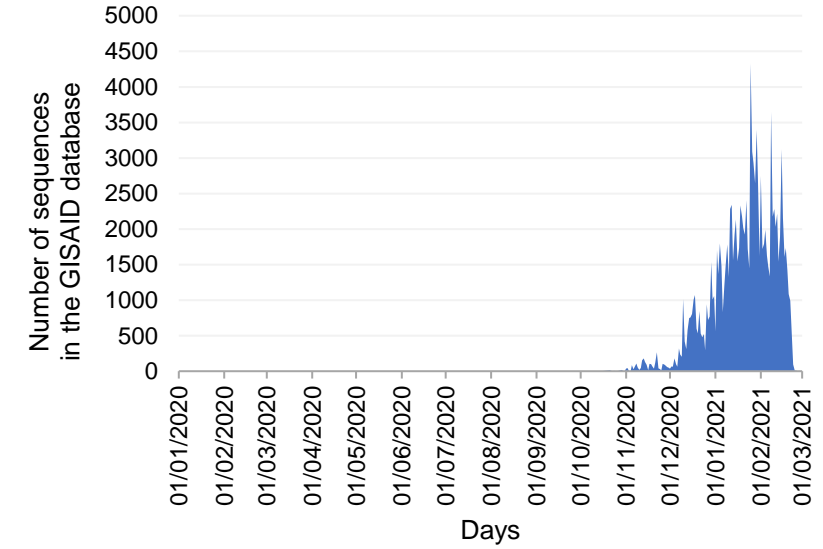
20H/501Y.V2
