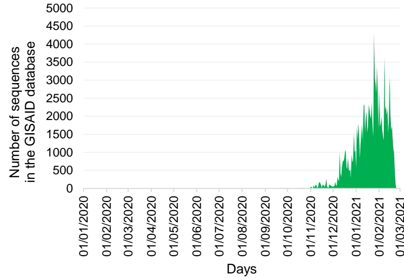
20I/501Y.V1
